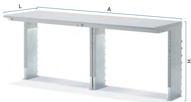
PIANO DI LAVORO CON TELAIO REGOLABILE DA 720 A 1138 mm
