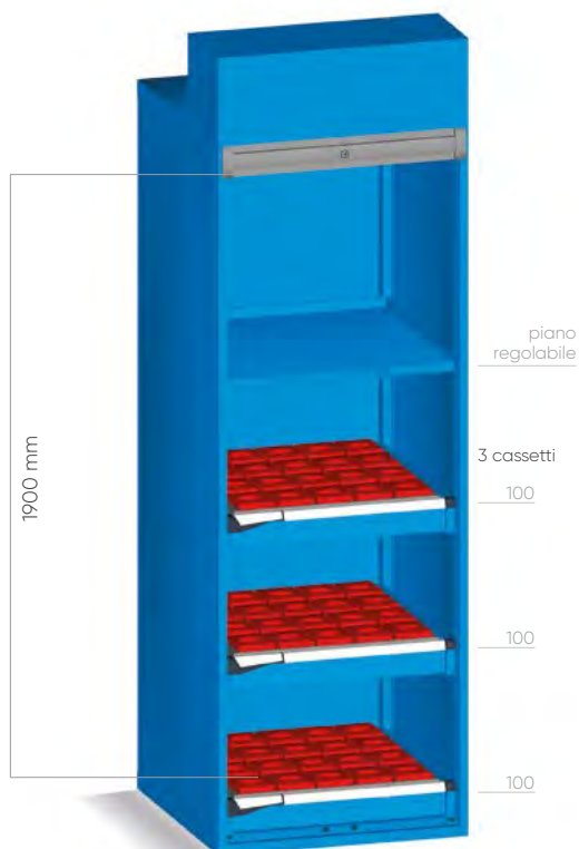
armadio con tapparella
