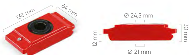
BOCCOLA HSK A32-B40
