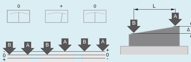
Misure differenziali con segni di polarità opposti (+A -B)
