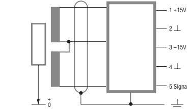
Schema del connettore DIN 5 poli
