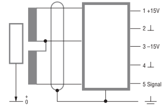
Schema del connettore DIN 5 poli
