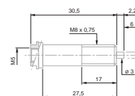
Pignone pneumatico per tastatori FMS
